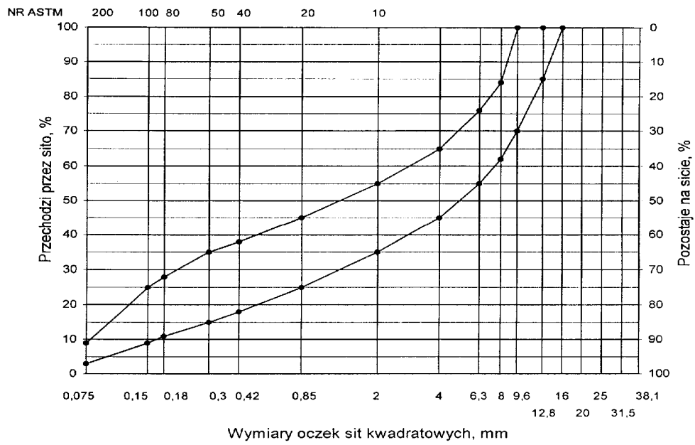
Rys. 6. Krzywe graniczne uziarnienia mieszanki mineralnej BA od 0 do 12,8 mm do warstwy wiążącej nawierzchni drogi o obciążeniu ruchem KR2
