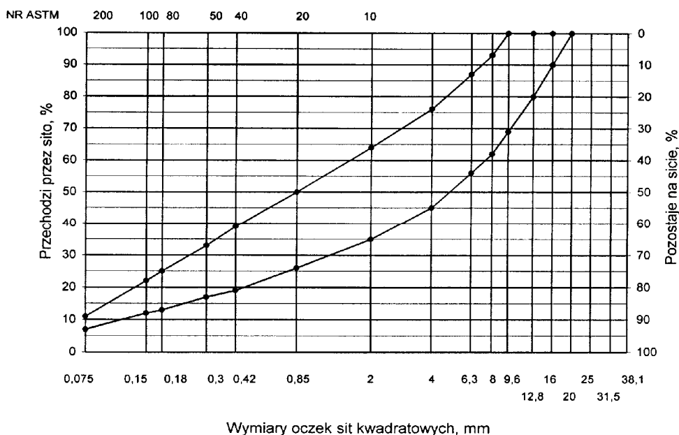
Rys. 1. Krzywe graniczne uziarnienia mieszanki mineralnej BA od 0 do 12,8 mm do warstwy ścieralnej nawierzchni drogi o obciążeniu lub KR-2
