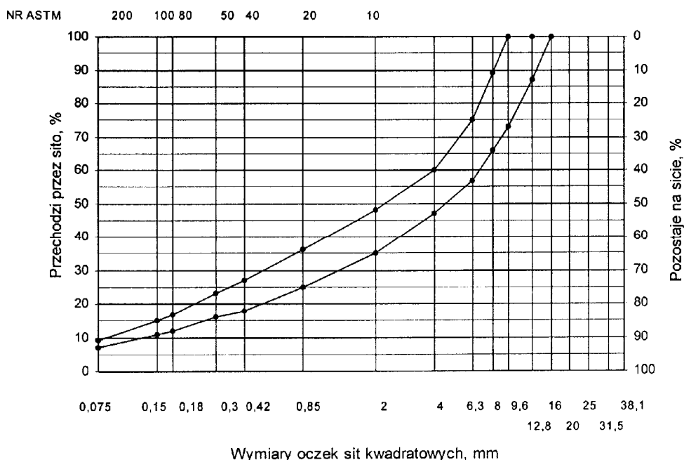
Rys. 2. Krzywe graniczne uziarnienia mieszanki mineralnej BA od 0 do 12,8 mm do warstwy ścieralnej nawierzchni drogi o obciążeniu ruchem od KR-3 do KR-6. Zaprojektowana mieszanka BA 0/12,8 powinna
