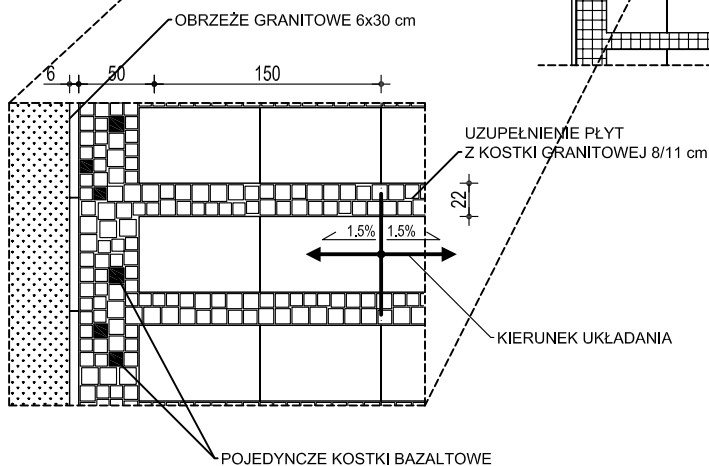
DETAL NAWIERZCHNI skala 1:50
