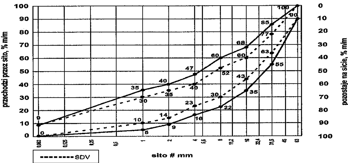
Rys. 2. Krzywe graniczne uziarnienia mieszanki kruszywa niezwiązanego 0/63 mm do warstw podbudowy
