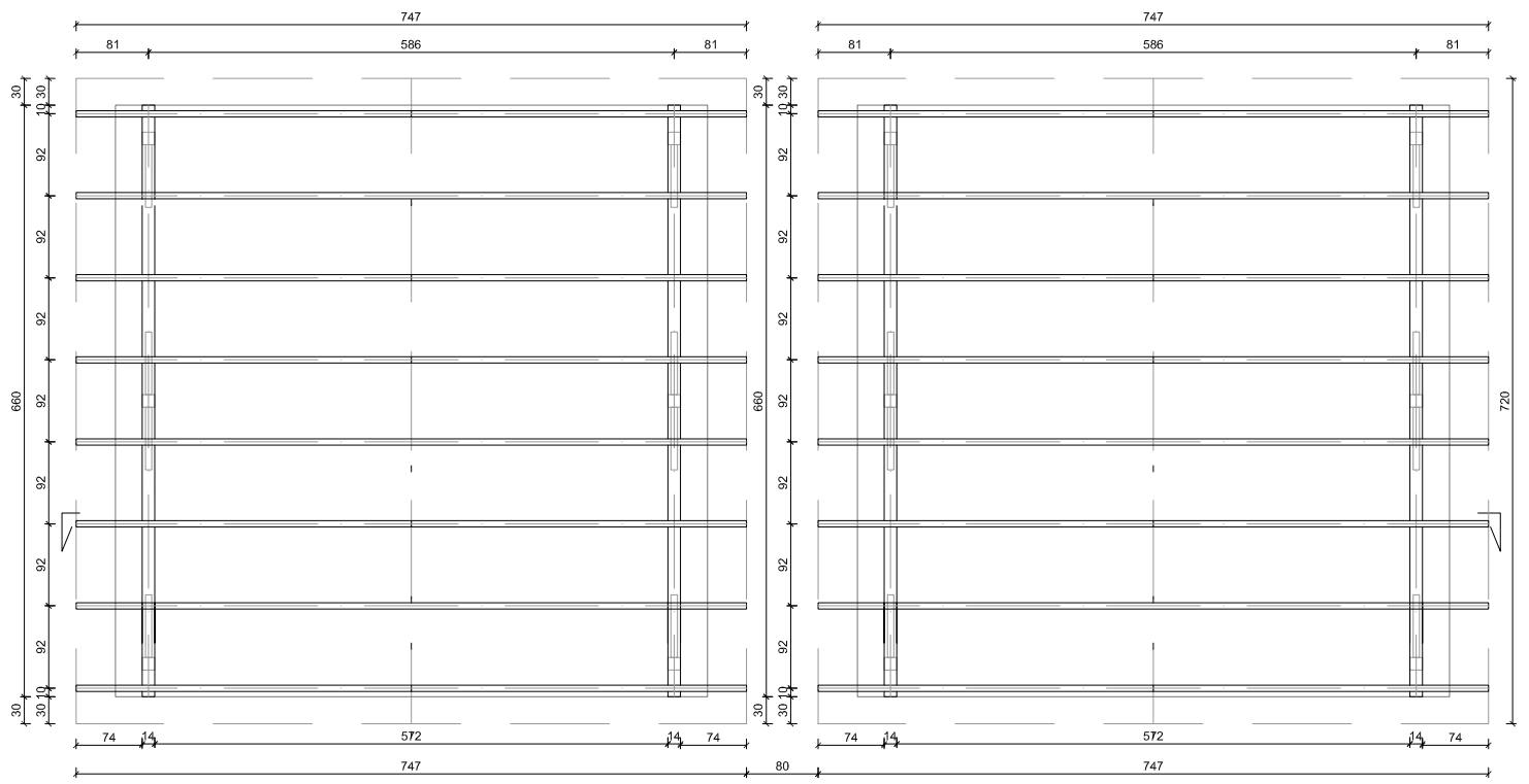
Rzut więzby
