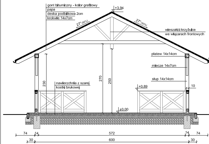
Przekrój poprzeczny
