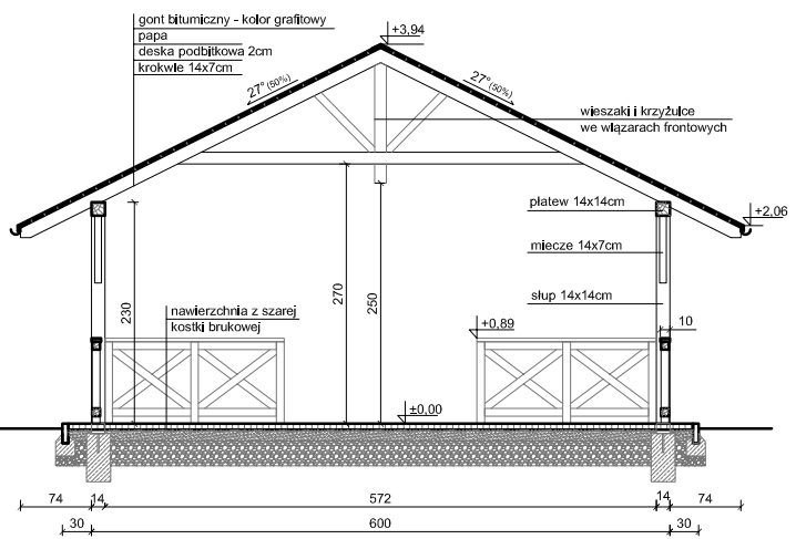
Przekrój poprzeczny
